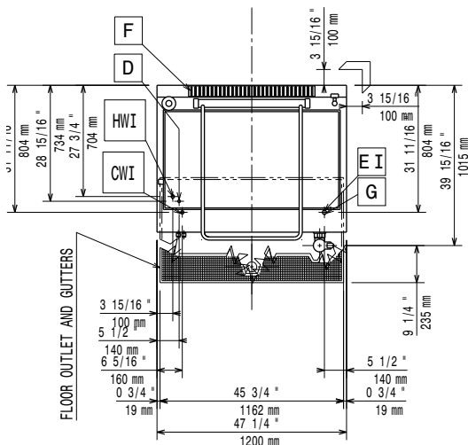
Felülnézet
